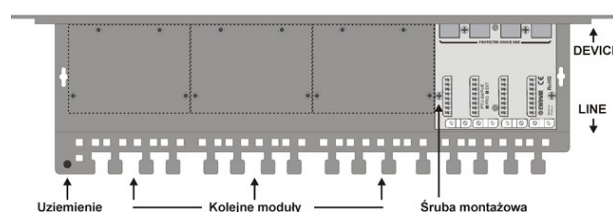
Názorná ukázka montáže modulů do krytu
