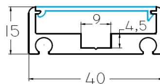
Standardní výztuha CPREG-S
