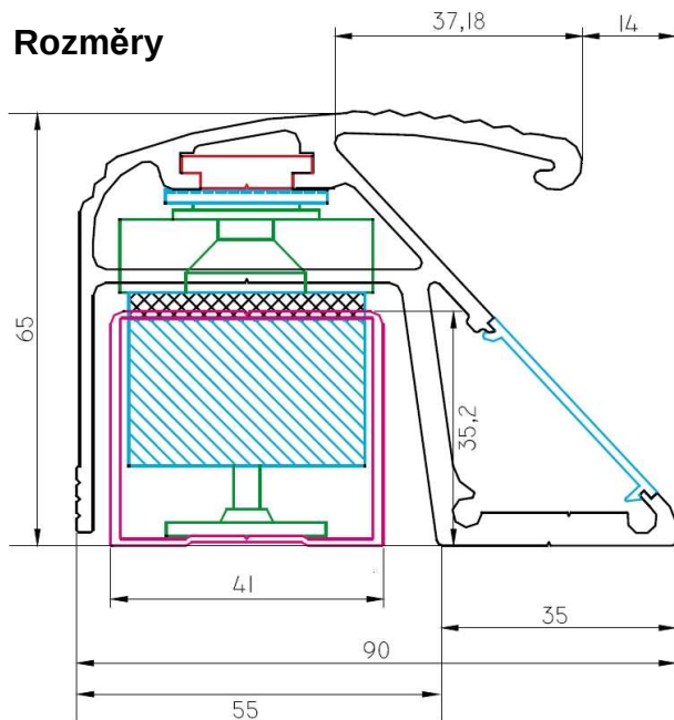
Hliníkový kryt CPREG-1
