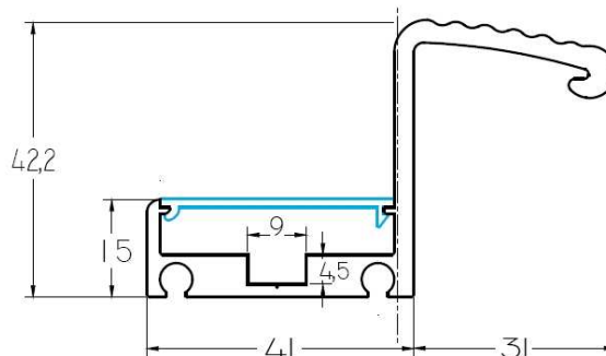
Výztuha s rukojetí CPREG-P
