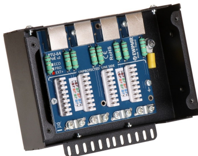
Názorná ukázka montáže modulů do krytu
